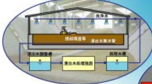
EX.5 散水洗浄方式
