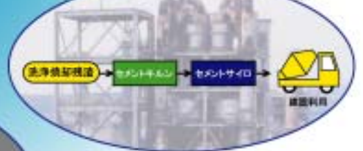
EX.7 洗浄灰のセメント原料利用
